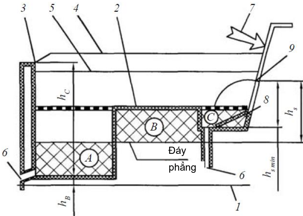
Hình 2/6.6 Hốc điều khiển nhiều mức
