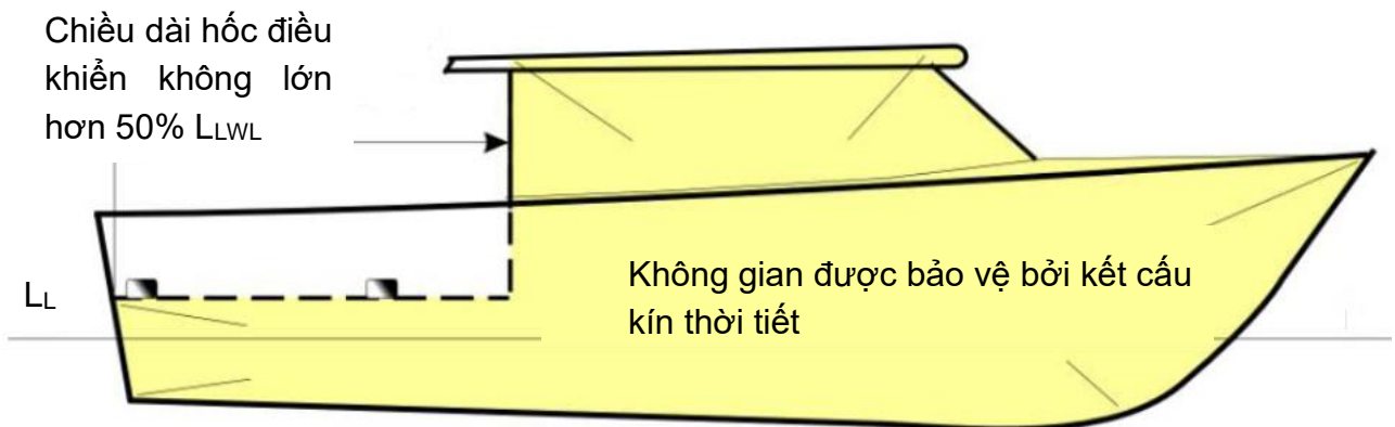
Hình 1/1 - Tàu có hốc điều khiển
