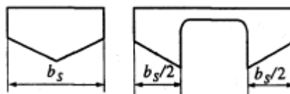
Hình 2/3.12 Chiều rộng của diện tích va đập đáy tàu tham chiếu
