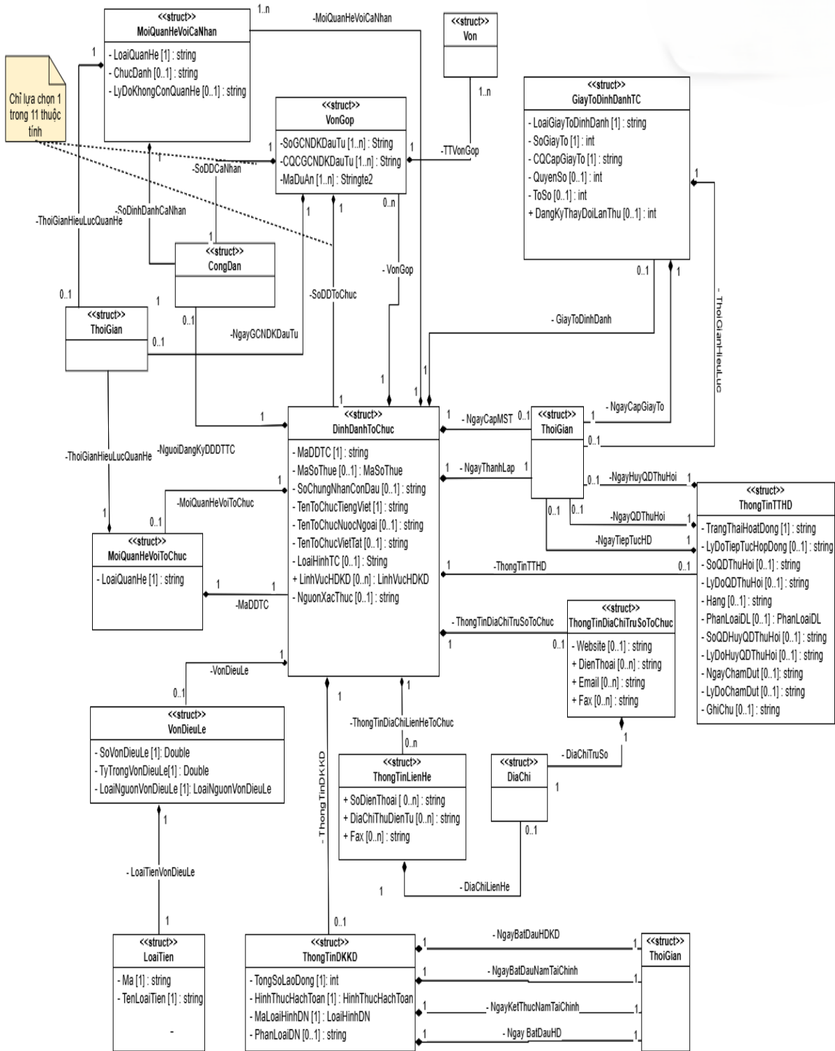
Hình A.2.2. Cấu trúc và mối quan hệ giữa các cấu trúc trong mô hình dữ liệu pháp nhân được mô tả bằng ngôn ngữ UML – Thông tin cơ bản về pháp nhân
