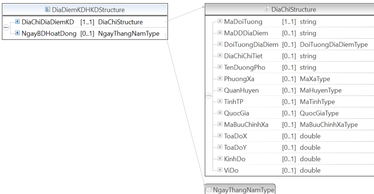
Hình C.1.74. Cấu trúc DiaDiemKDHKD
